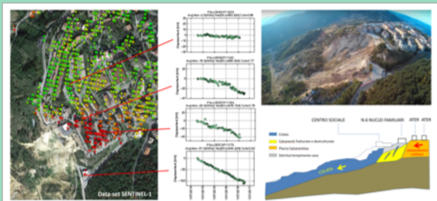
▲ Figura 3: Permanent Scatterers individuati a monte della frana complessa di Stigliano e modello schematizzato del fenomeno franoso
